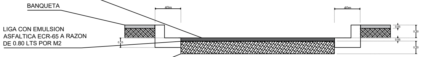
DETALLE CORTE TRANSVERSAL
